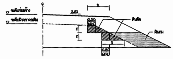
รูปตัดการก่อสร้างลาดคันทางบนถนนเดิม งานตัดไม้ (งานขุดดิน, งานตัดหิน, งานตัดดินแข็ง และงานขุดอื่น ๆ)
